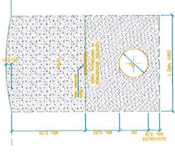
KESİT B-B
